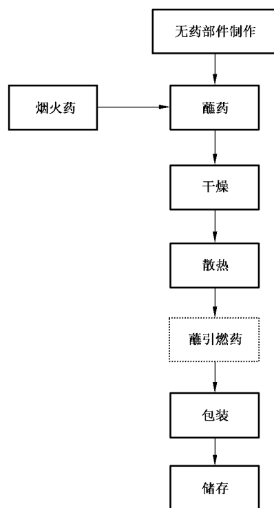
图 A. 14 线香类(涂敷型)生产流程图
