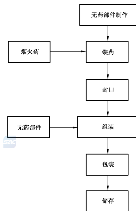
图 A.21 线香(包裹药型)类生产流程图
