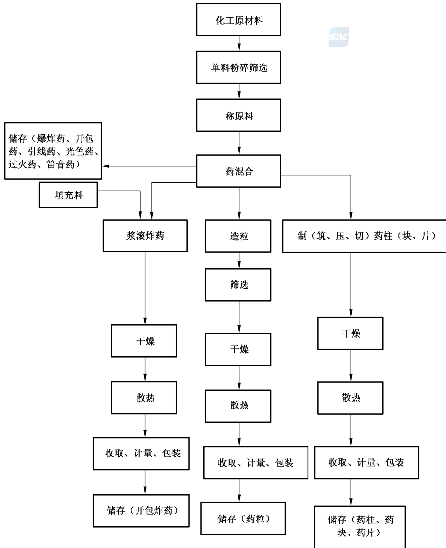
图 A.2 药物裸药效果件生产工艺流程图 [炸药、开包药、药粒、药柱(块、片)、引线药、光色药、过火药、笛音药]
